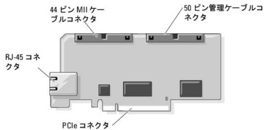
図 1-1. DRAC 5 ハードウェア機能
